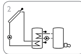
Zonnestelsysteem met naverwarming (pagina 11)
