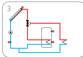
Standard-Solaranlage mit Überwärmefuhr (Seite 14)
