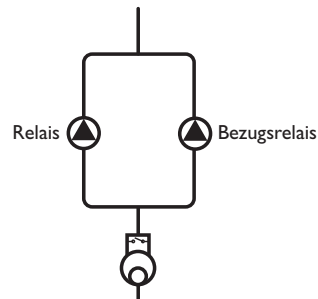
Beispielschema für Zwillingspumpen mit vorgelagertem Volumenmessteil
