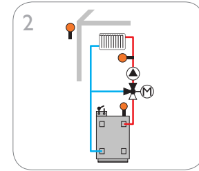
1 gemischter Heizkreis mit Nachheizung (Anforderung) (siehe Seite 15)
