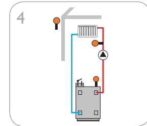
1 ungemischter Heizkreis mit Nachheizung (Anforderung) (siehe Seite 17)
