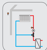
1 gemischter Heizkreis mit externer Wärmequelle (z. B. Fernwärme)
