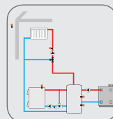
1 gemischter Heizkreis mit Festbrennstoffkessel und Nachheizung (Anforderung)
