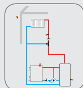
1 gemischter Heizkreis mit Festbrennstoffkessel
