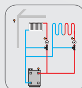
2 gemischte Heizkreise mit Nachheizung (Anforderung)
